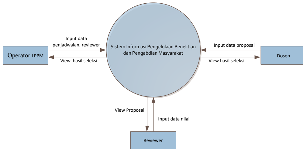
Gambar 3. Diagram Konteks
