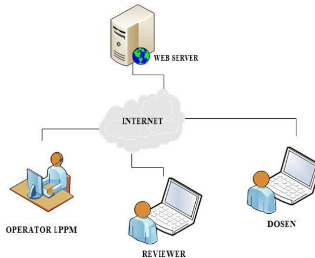
Gambar 2. Arsitektur Pengguna
