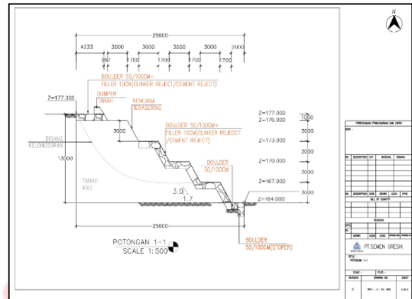
Desain Potongan 1-1
