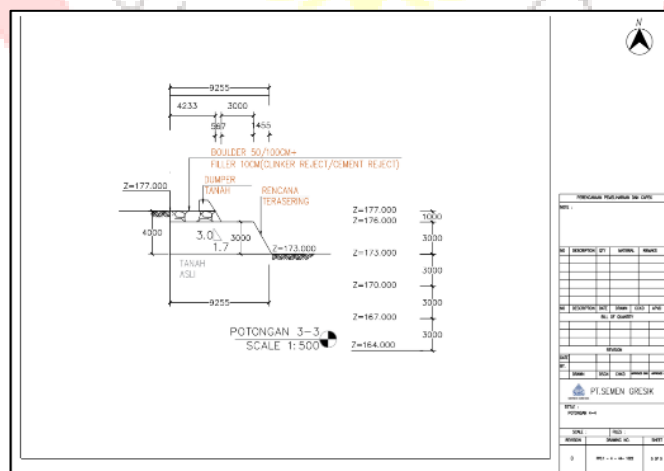
Desain Potongan 4-4
