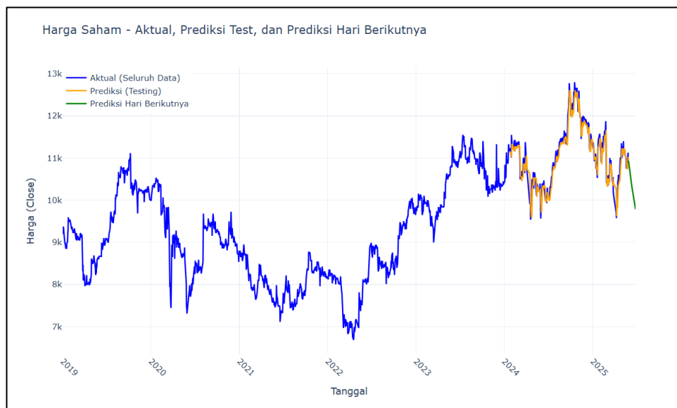
Grafik Hasil Prediksi RNN 30 Hari
